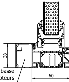
C-C ( 1/2 )
