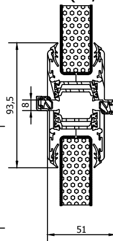
C-C ( 1/2 )
