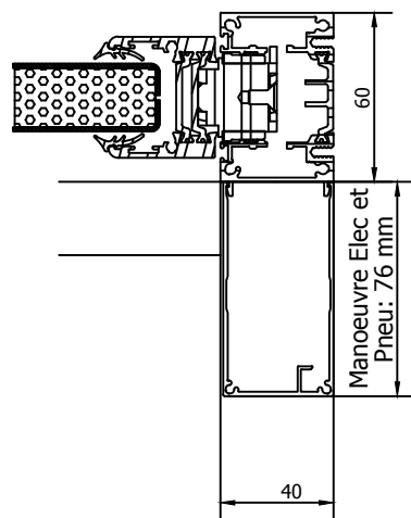
C-C ( 1/2 )
